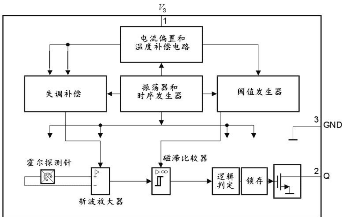
四、功能框图:
