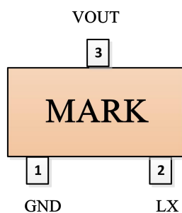
SOT23
